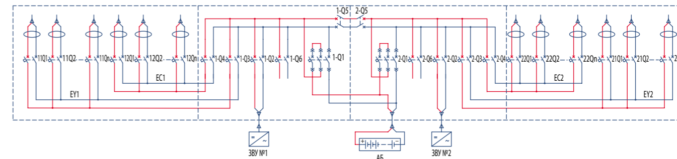
Схема СОПТ ExOnSys-XL-1-УХЛ4
