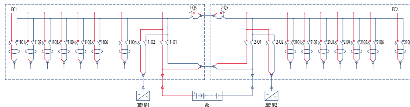
Схема СОПТ ExOnSys-M-2-UX14
