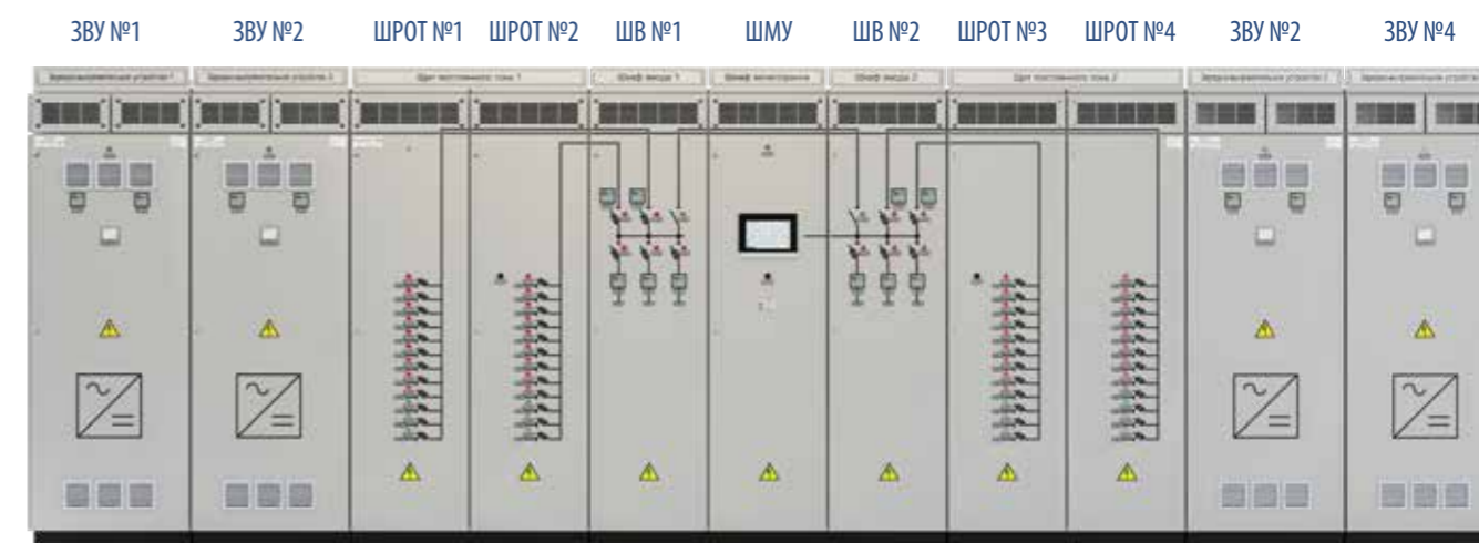
Рис. 7. Пример внешнего вида СОПТ «ExOnSys-XL-2»
